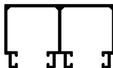
Trilho superior SD 22
